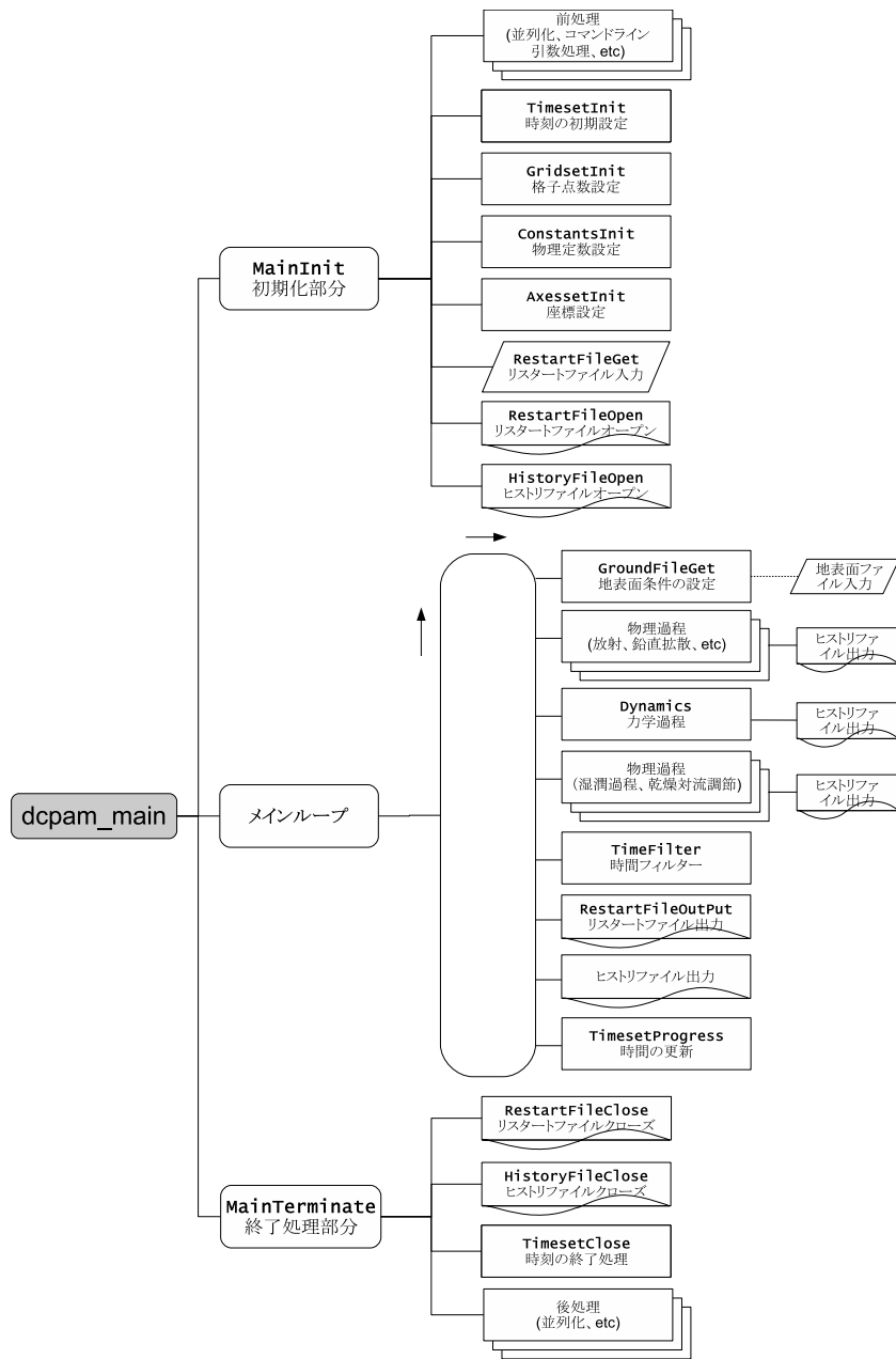
図 2.1: dcpam5-primitive の構造の概要. アルファベット太字で書かれているのはメインプログラム dcpam_main (dcpam.main.F90) 中で呼ばれているサブルーチンである. 骨格を把握する上で冗長なものはひとまとめにしてあり, 個別のサブルーチン名は記載していない. MainInit および MainTerminate はメインプログラムファイル中に内部副プログラムとして定義されるサブルーチンである. 破線は, メインループの初回でのみ呼ばれることを示す. 図中では, 地表面ファイル入力とその一例として示されている. 診断量であるヒストリデータは, その出力の初期化と終了処理は主プログラムの MainInit および MainTerminate で行い, 出力自体は各所で行う.
