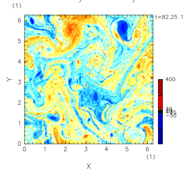
lower layer Vorticity
