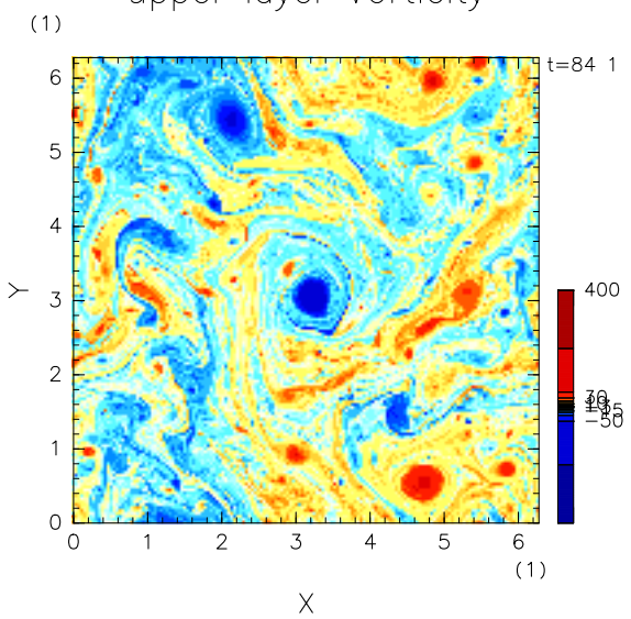
upper layer Vorticity
