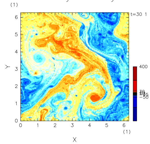
lower layer Vorticity
