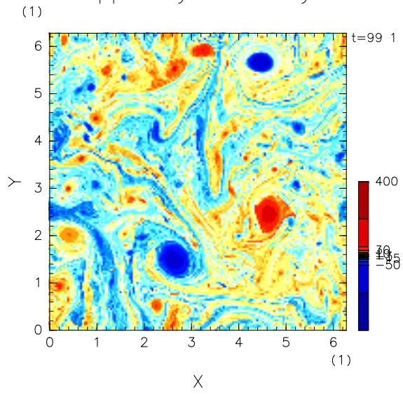
upper layer Vorticity
