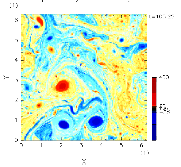
upper layer Vorticity
