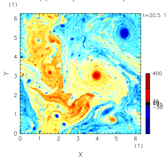
upper layer Vorticity
